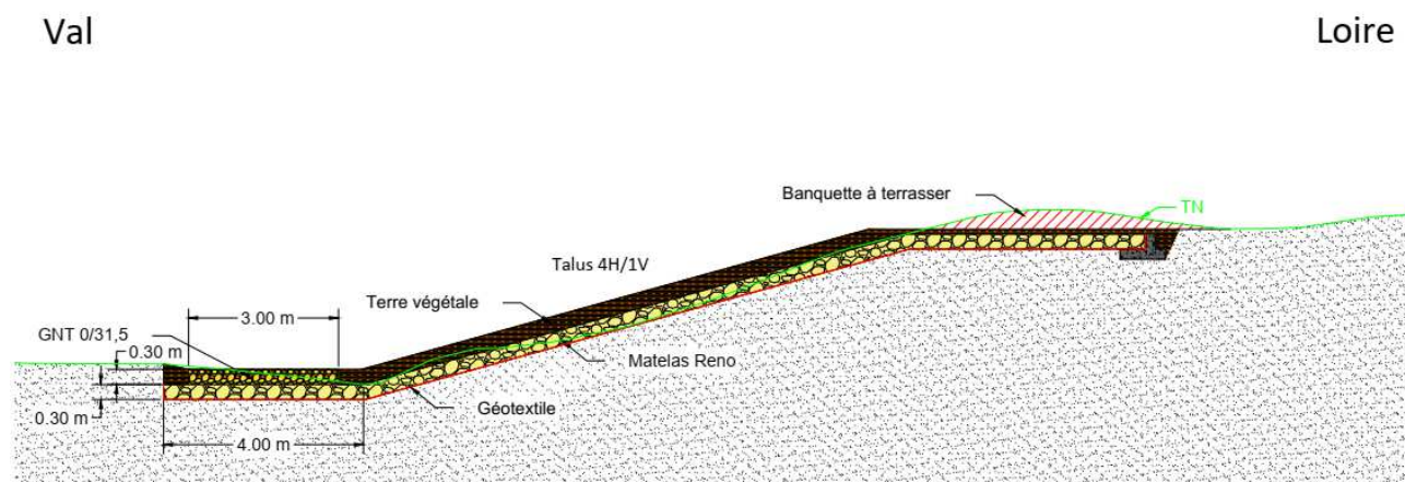
Travaux de fiabilisation à la surverse – Coupe type
