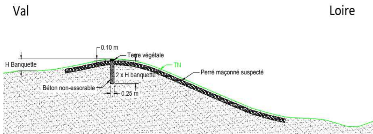
Travaux de fiabilisation de la banquette côté Loire – Coupe type
