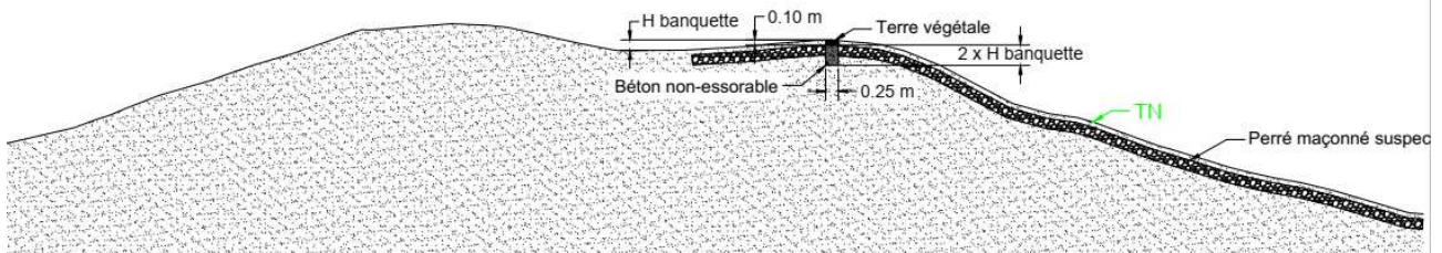
Travaux de fiabilisation de la banquette coté Val - Coupe type
